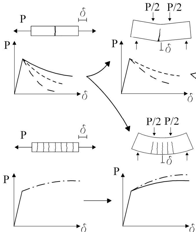
Figura 2: Risposta meccanica di strutture caratterizzate da capacità redistributive differenti: trazione uniassiale e flessione.
