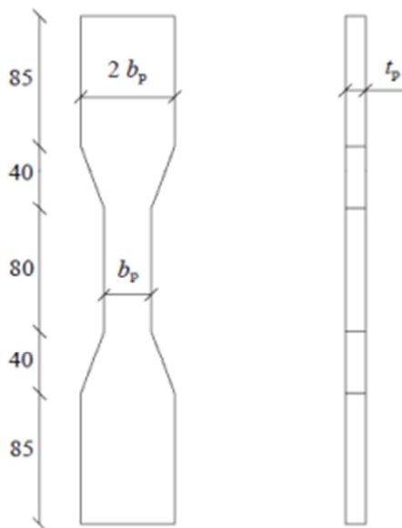
Fig. A1 – Geometria del provino (misure in mm).
