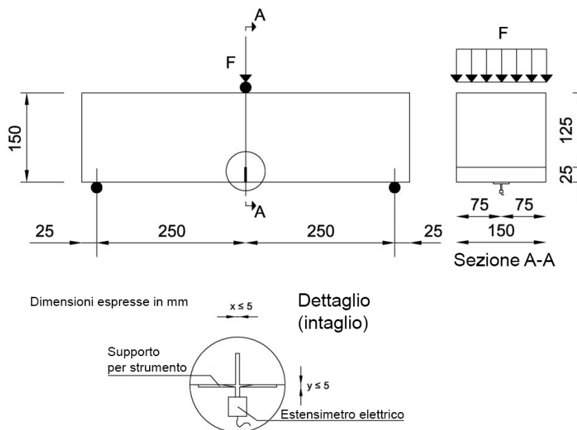
Figura 3: Geometria del provino per la caratterizzazione a flessione (EN 14651)
