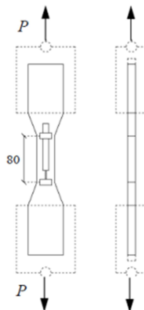
Fig. A2 – Strumentazione per la prova di trazione (misure in mm).
