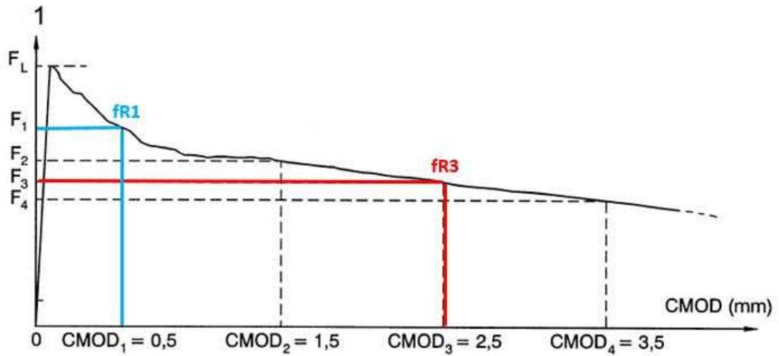
Figura 4: Tipica curva di una prova di flessione condotta secondo la EN 14651.
